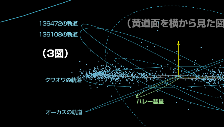
(黄道面を横から見た図)
