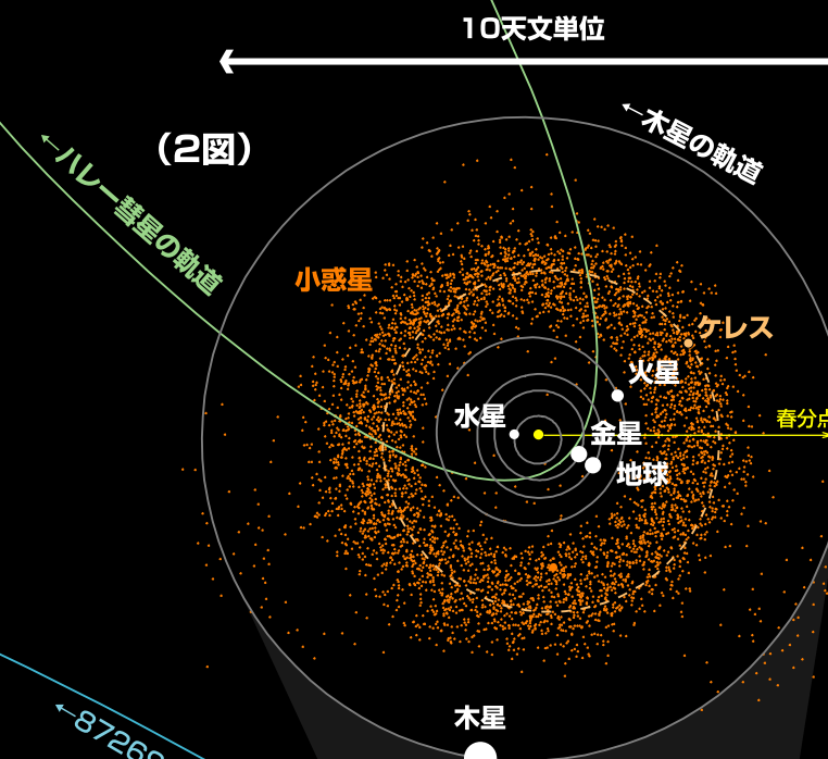
(黄道面を上から見た図)
